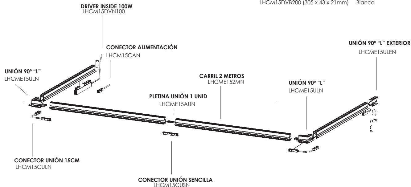
DRIVER INSIDE 100W DC48V / 200W LHCM15DVN100 (225 x 41 x 21mm) Negro LHCM15DVB100 (225 x 41 x 21mm) Blanco LHCM15DVN200 (305 x 43 x 21mm) Negro LHCM15DVB200 (305 x 43 x 21mm) Blanco
