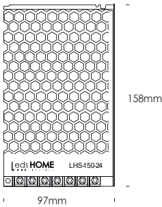
FUENTE DE ALIM. 150W
